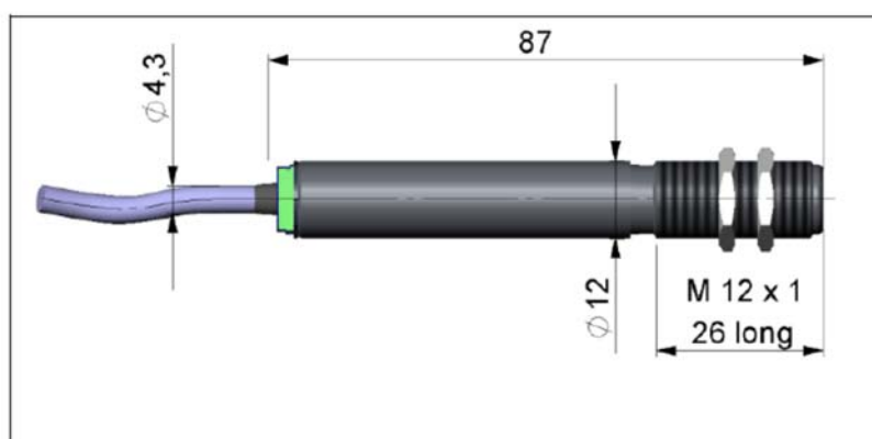
Dimensions TIN-SS
